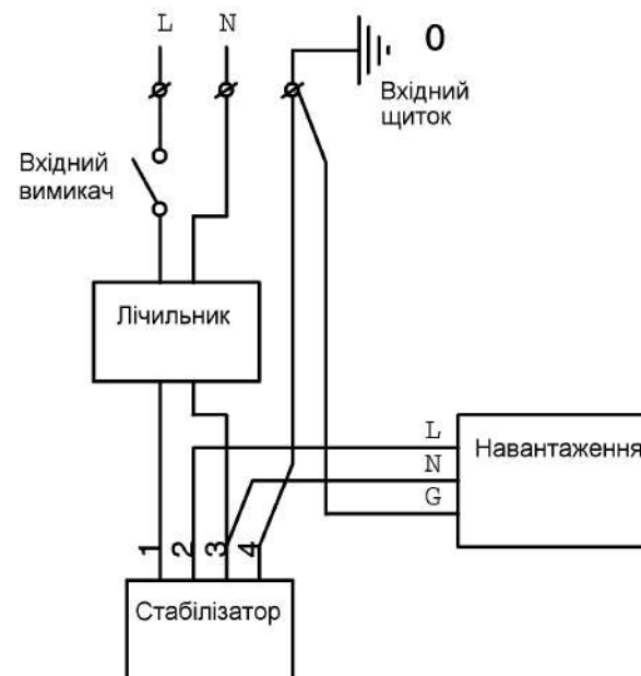
Схема підключення стабілізатора до однофазної мережі.
